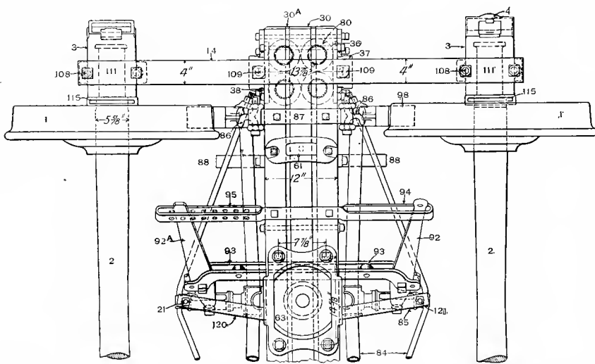
Fig. 4581. Part Plan.
